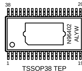
TSSOP38 TEP
